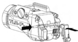
Schalter umbauen
